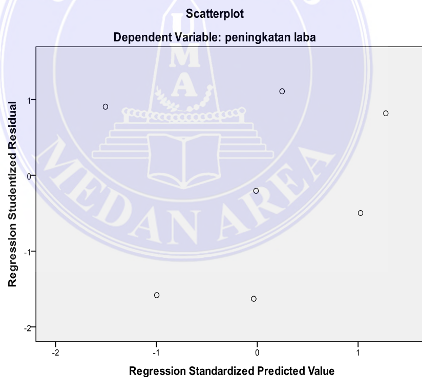
Gambar 4.2 : Grafik Sccatterplot
