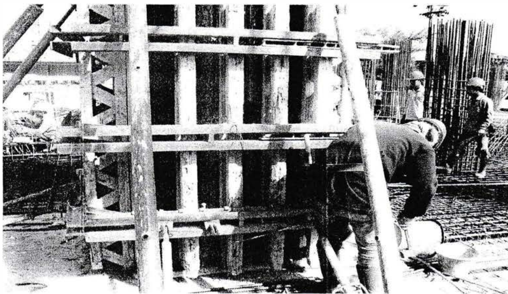
Gambar 2.10.4 Bekisting
