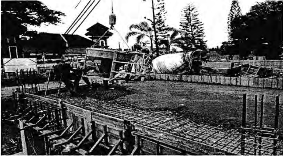
Gambar 3.13 Pengecoran Plat Lantai
