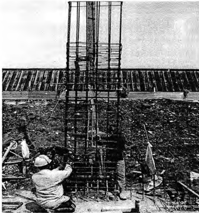
Gambar. Tulangan Kolom Yang Sudah Berdiri Lokasi : Jalan william iskandar, Pancing
