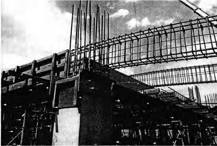
Gambar 3.19 Tulangan balok
