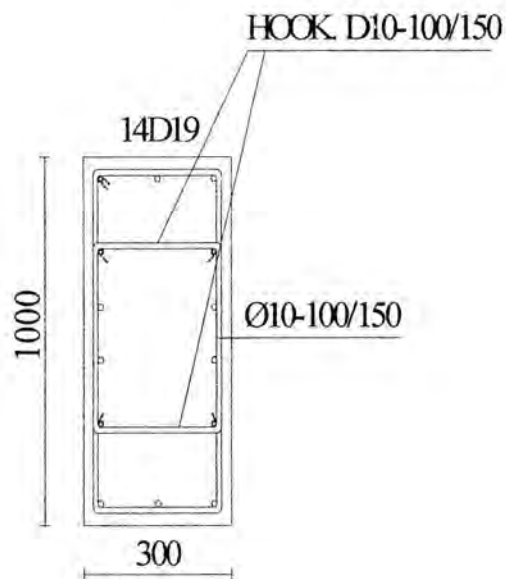
Gambar 4.1 Detail kolom K2 (1000 x 300) mm
