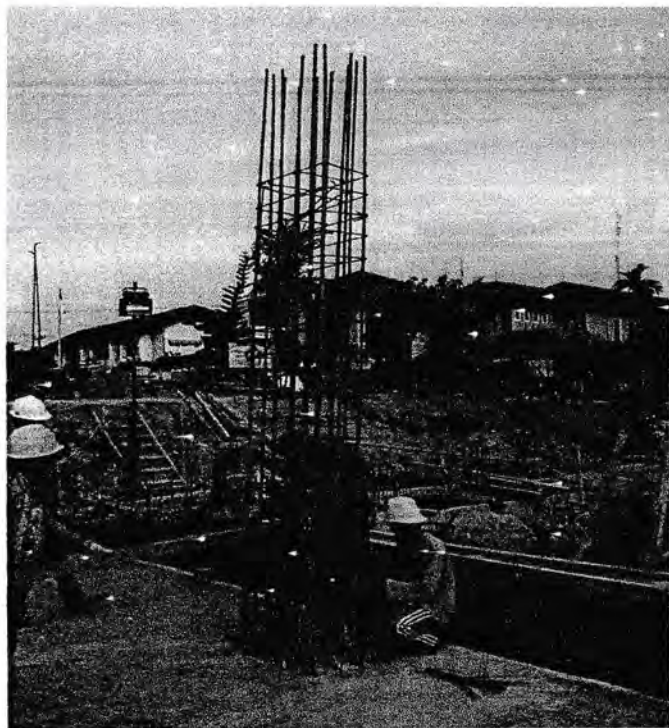
Gambar Rangkaian Kolom Lokasi : Jalan william iskandar, Pancing
