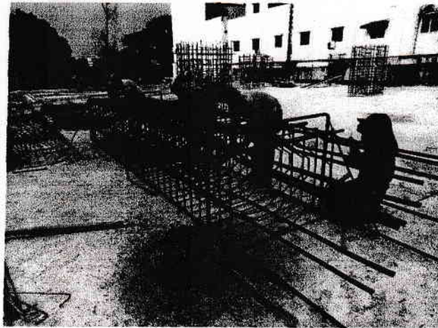
Gambar 2.23 Penulangan Kolom
