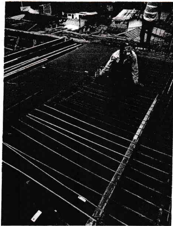
Gambar 2.25 (d) Pemasangan bekisting
