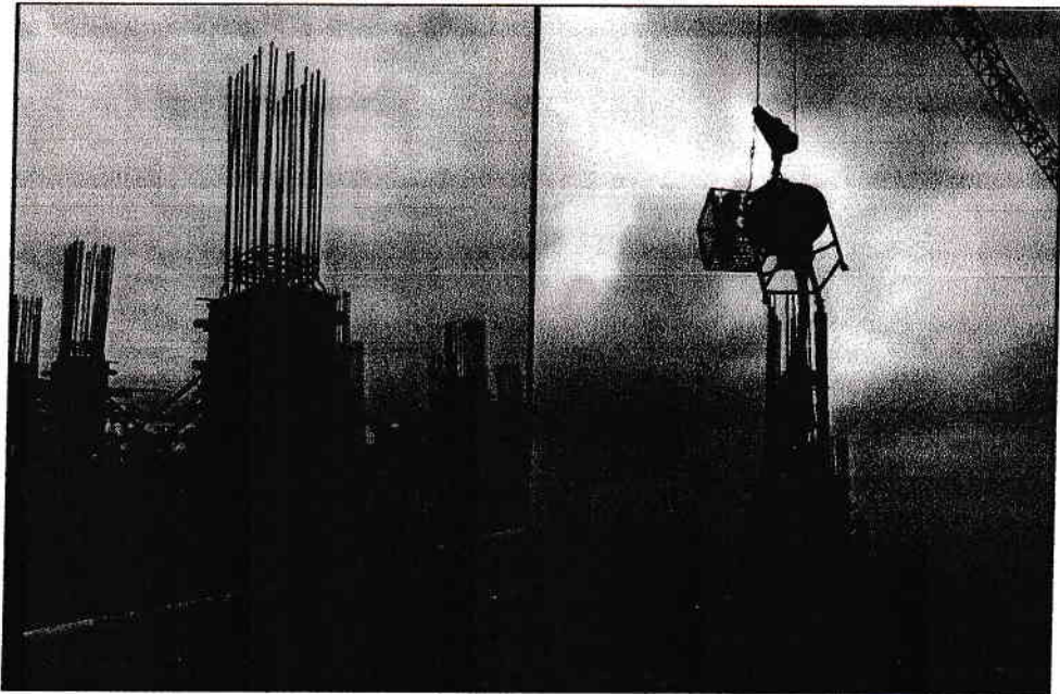
Gambar 2.24 Pemasangan bekisting dan pengecoran
