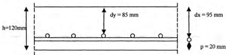
Gambar 4.4 Penulangan Pelat lantai
