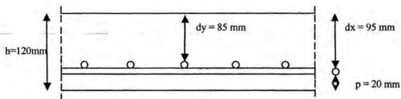
Gambar 4.2 Penulangan Pelat lantai
