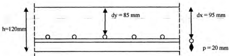
Gambar 4.8 Penulangan Pelat lantai
