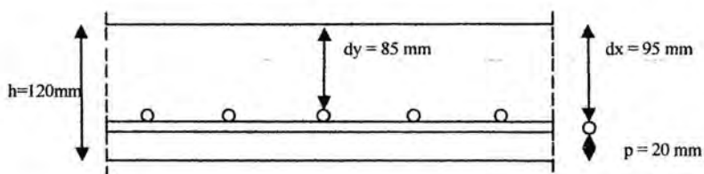
Gambar 4.6 Penulangan Pelat lantai
