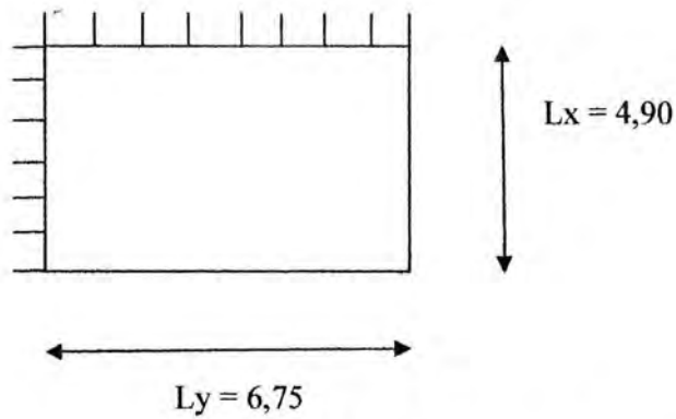
Gambar 4.5 Pelat Lantai tipe III
