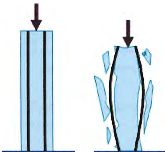
Gambar 2.6 Ilustrasi Tulangan kolom tanpa sengkang
