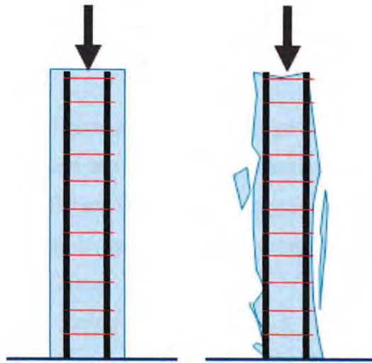
Gambar 2.7 Tulangan kolom pakai sengkang
