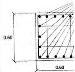
DETAIL K1 SKALA 1 : 20
