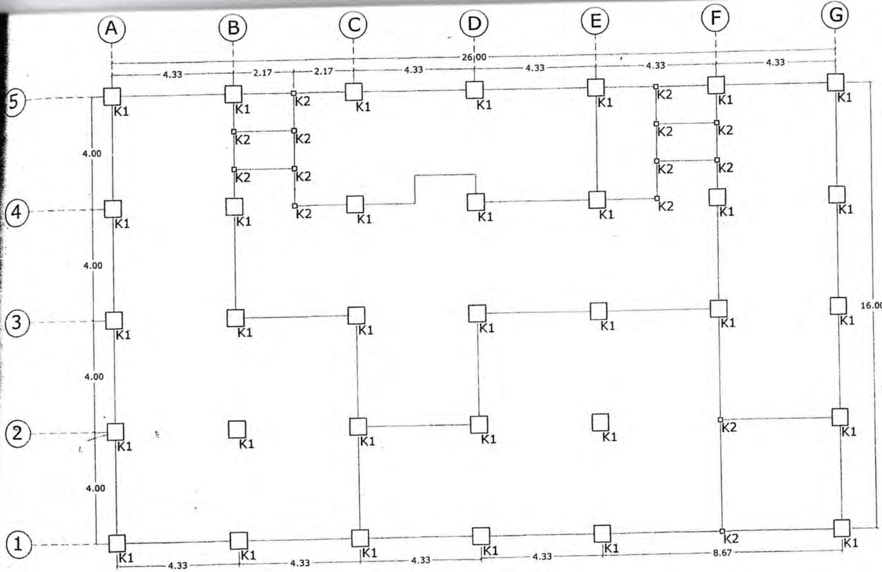
DENAH KOLOM LANTAI 3 SKALA 1 : 100
