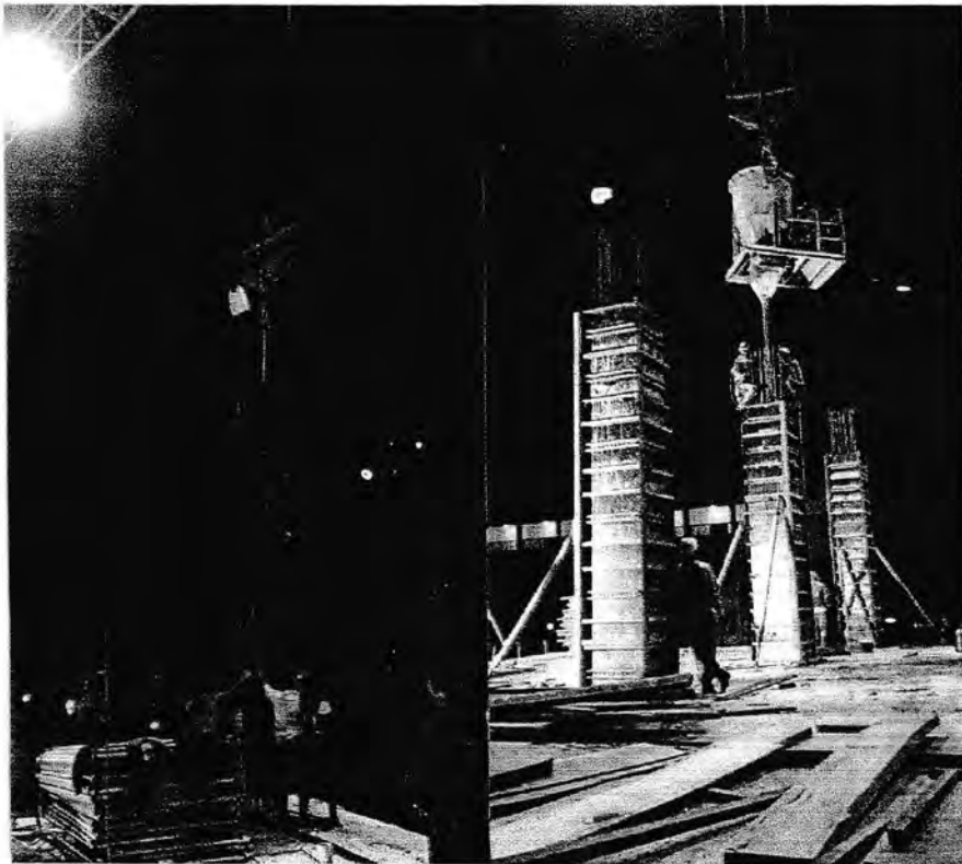
Pemasangan Besi Tulangan Kolom dan Pengecoran
