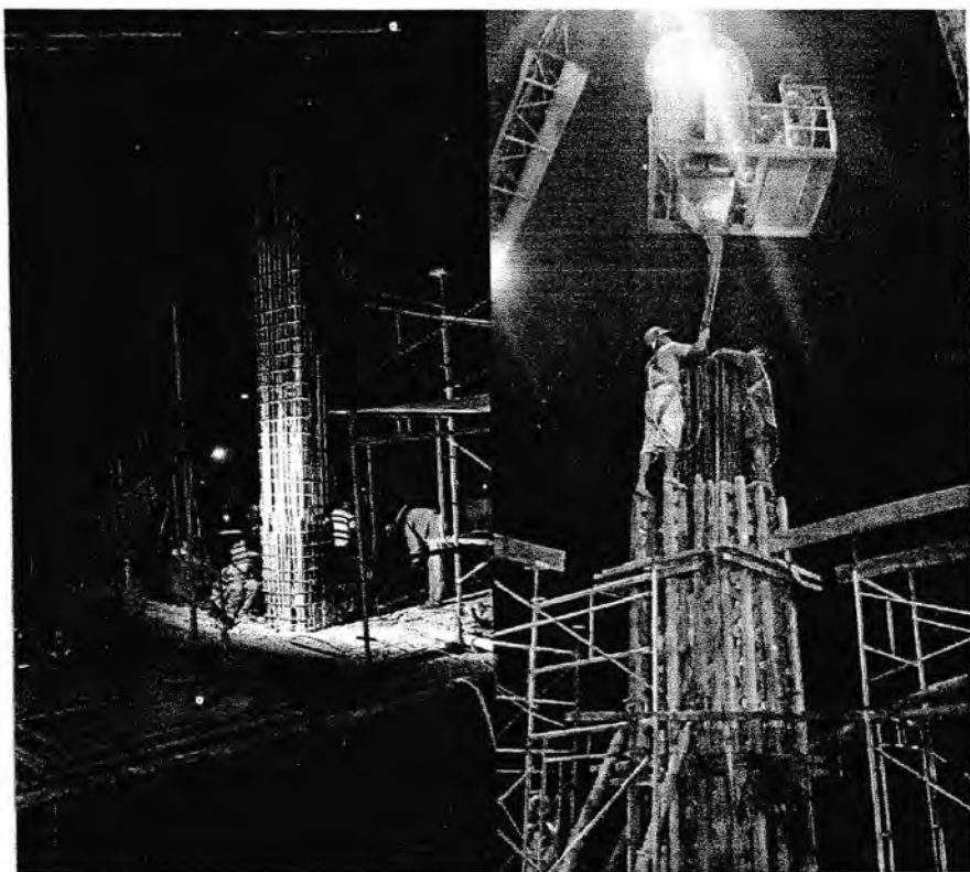
Penyambungan dan Pengelasan Besi Tulangan Kolom
