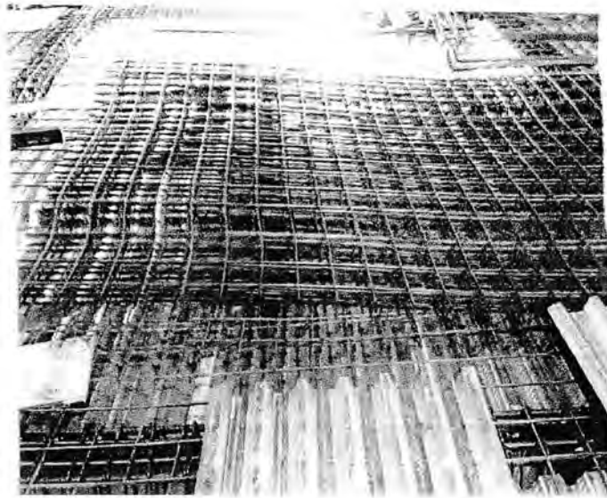
Gambar 3.7. Tulangan plat lantai
