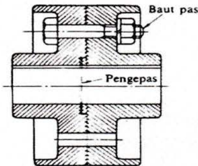
Gbr.2.1. Kopling Flens Kaku
