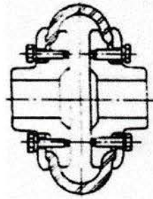
Gbr.2.4. Kopling Karet Ban
