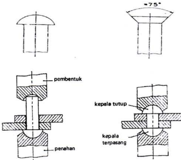
Gambar 3.7. Paku Keling
