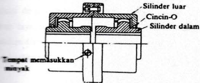
Gbr.2.7. Kopling Gigi
