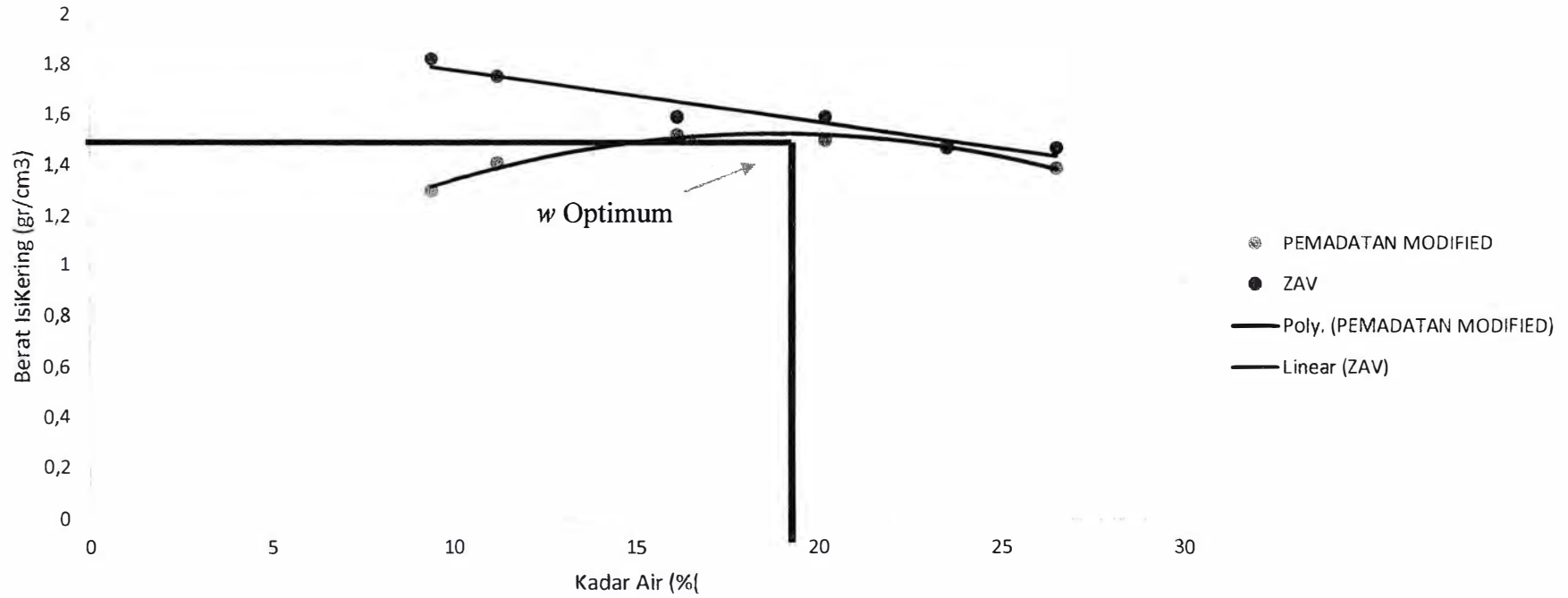
Grafik Pemeriksaan Kepadatan Standart
