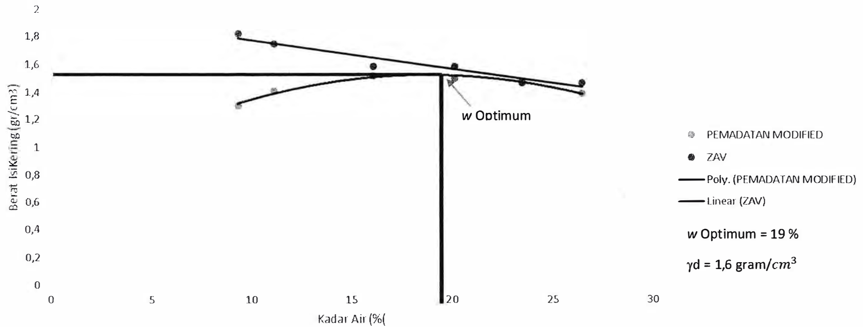
Grafik Pemeriksaan Kepadatan Berat (modified)
