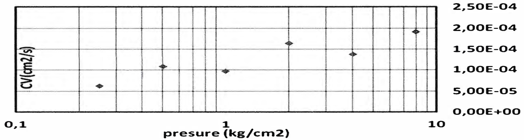
grafik persure Vs Cv
