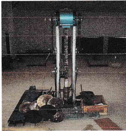
Gambar IV.1 Mesin Sondir
