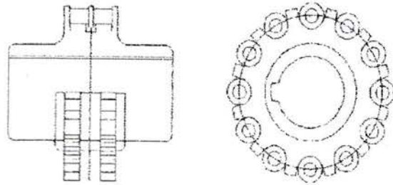
Gambar. 2.8. Kopling Rantai
