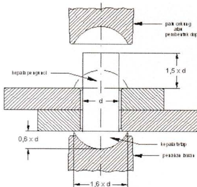
Gambar. 3.7. Paku Keling
