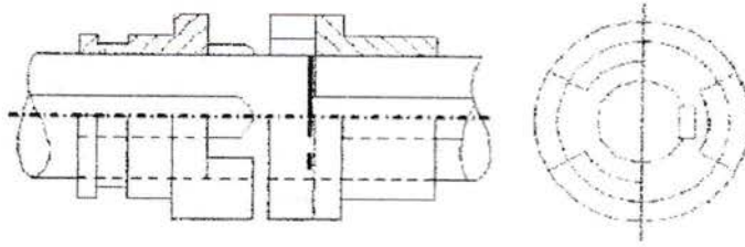
Gambar. 2.10. Kopling Cakar
