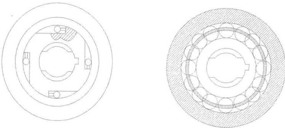
Gambar. 2.13. Kopling Friwil
