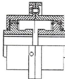
Gambar. 2.7. Kopleng Gigi
