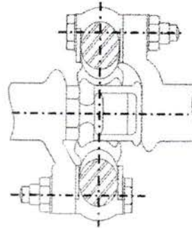
Gambar. 2.6. Kopleng Karet Bintang
