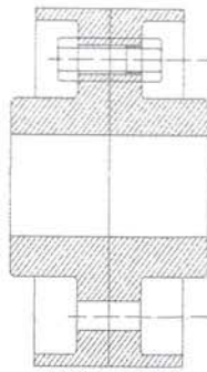
Gambar. 2.2. Kopling Flens Kaku
