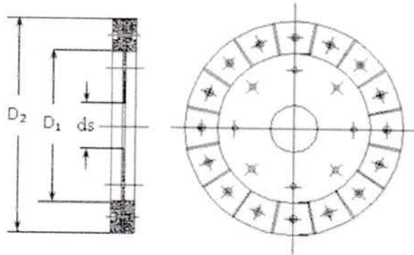
Gambar. 3.3. Kopleng plat
