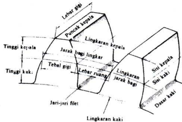
Gambar.3.1.Roda Gigi
