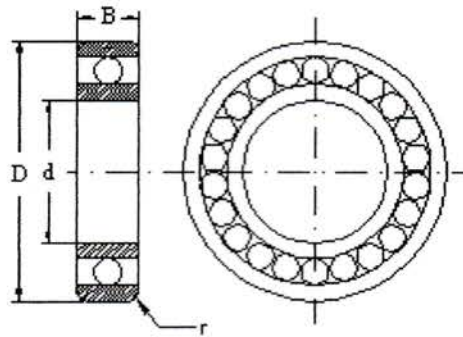
Gambar. 3.4. Bantalan gelinding
