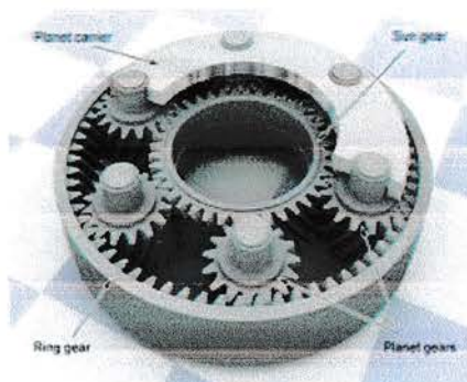
Gambar. 2.4. Roda gigi dalam dan pinyon
