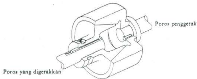
Gambar 2.11. Kopling Kerucut
