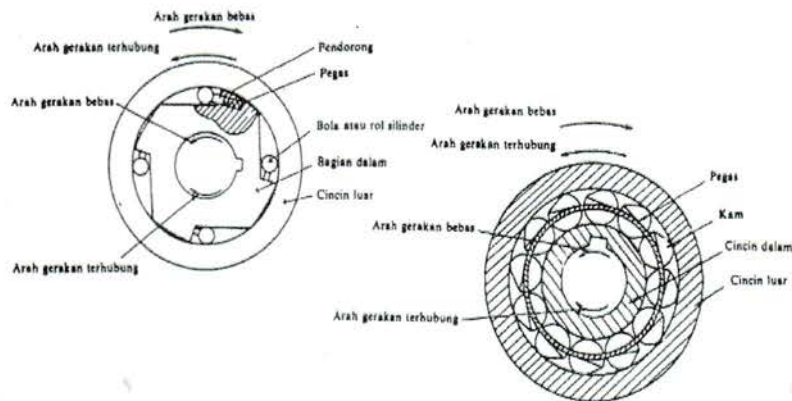
Gambar 2.13. Kopling Friwil
