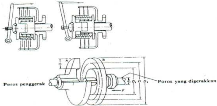
Gambar 2.12. Kopling Plat
