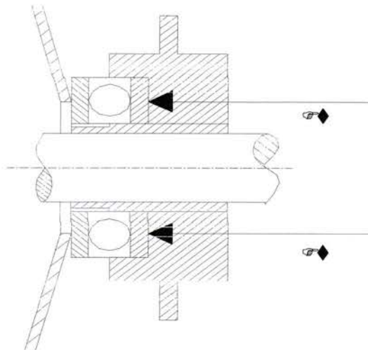
Gambar 10. 4. Bantalan Pembebas
