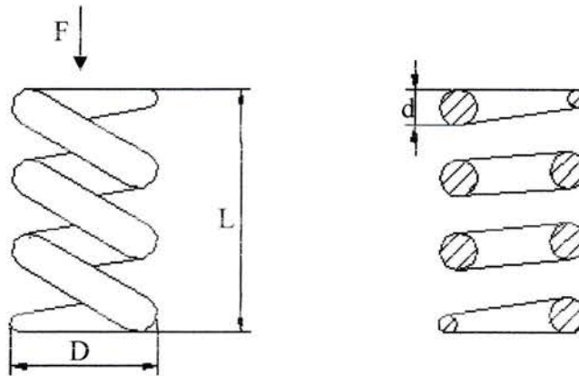
Gambar 8. 3. Pegas Kejut
