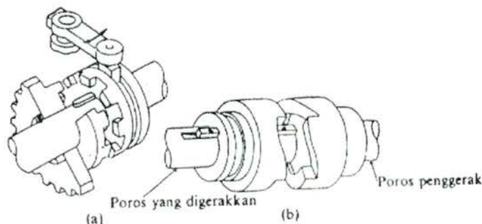
Gambar 2.10. Kopling Cakar
