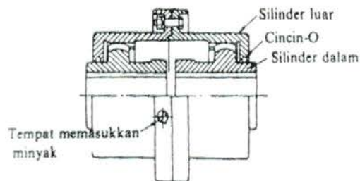
Gambar 2.7. Kopling Gigi
