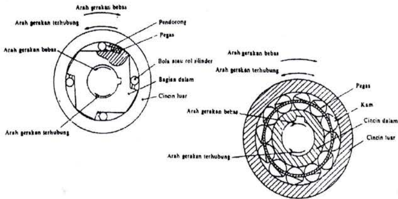
Gambar 2.13. Kopling Friwil
