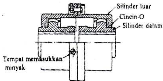
Gambar 2.7. Kopling Gigi
