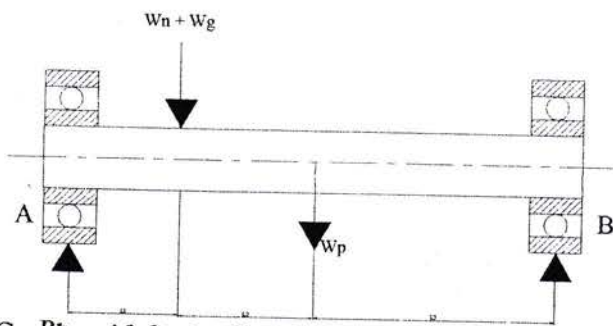
Gambar 10.2. Analisa Gaya Pada Bantalan Pendukung Poros
