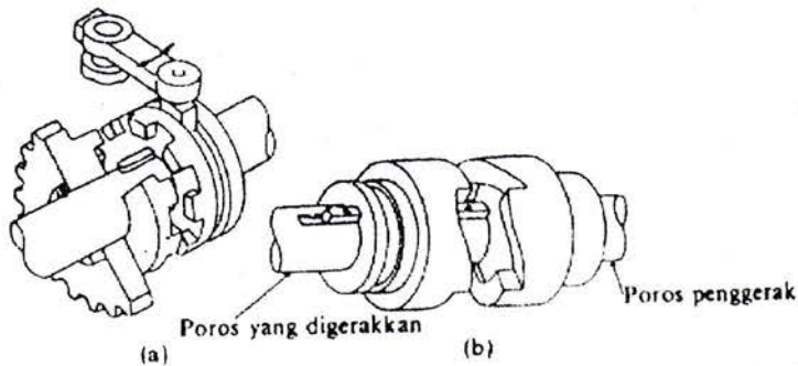
Gambar 2.10. Kopling Cakar
