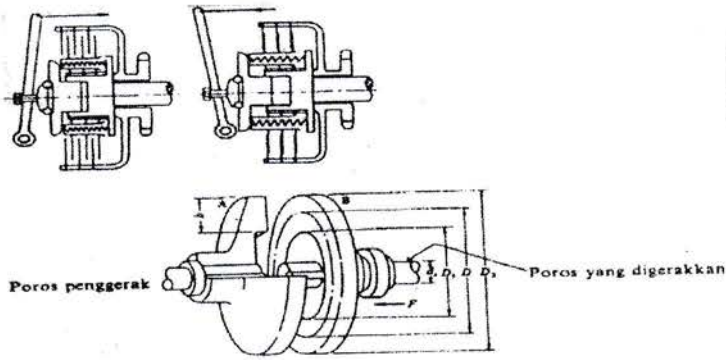
Gambar 2.12. Kopling Plat
