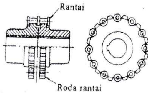
Gambar 2.8. Kopling Rantai
