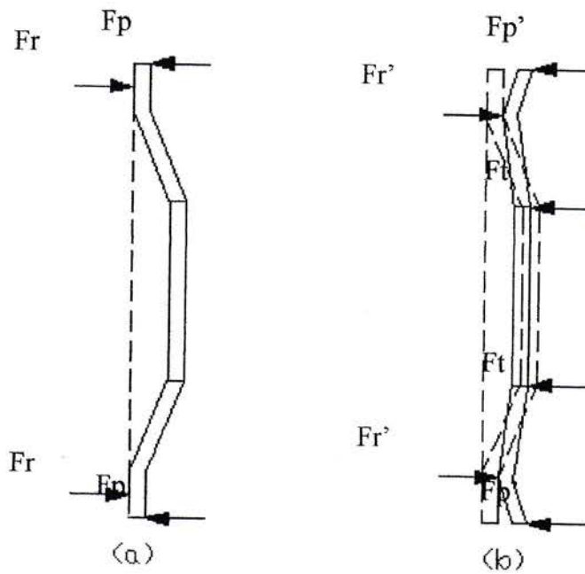
Gambar 8. 2. Diagram gaya-gaya yang bekerja pada pegas
