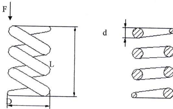
Gambar 8. 3. Pegas Kejut
