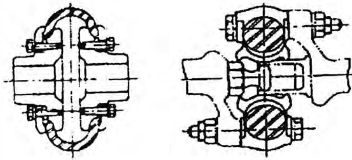
Gambar 2. Kopling Karet Ban dan kopling karet bintang
