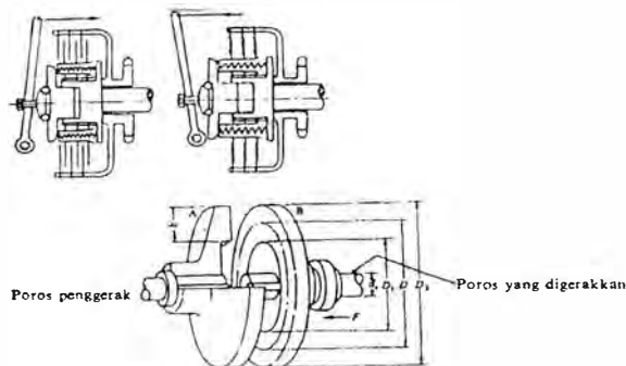
Gambar. Kopling Plat
