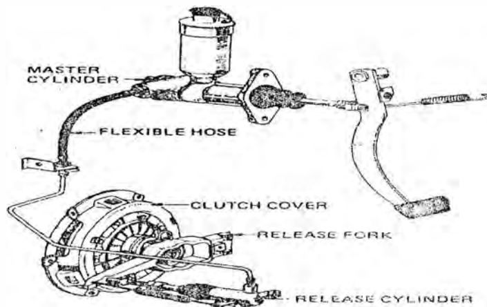
Gambar. Kopling Sistem Mekanis
