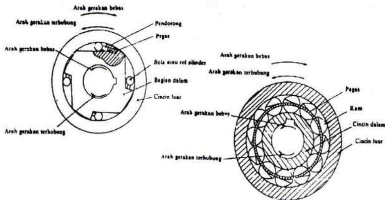
Gambar 2.13. Kopling Friwil
