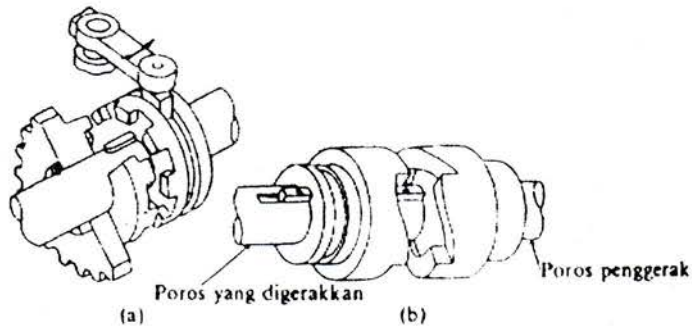
Gambar 2.10. Kopling Cakar
