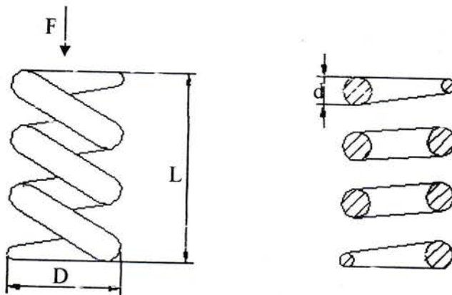
Gambar 8. 3. Pegas Kejut
