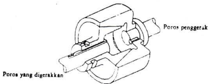
Gambar 2.11. Kopling Kerucut
