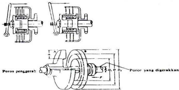
Gambar 2.12. Kopling Plat
