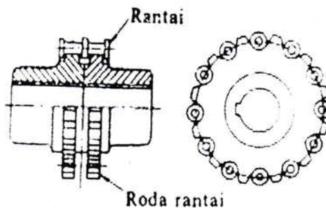
Gambar 2.8. Kopling Rantai
