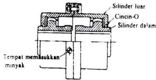
Gambar 2.7. Kopling Gigi
