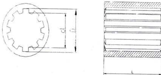
Gambar 5. 1. Naaf
