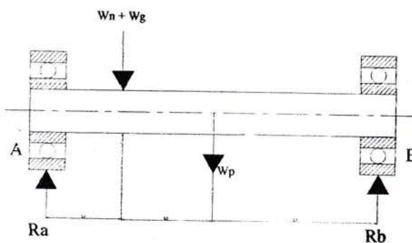
Gambar 10.2. Analisa Gaya Pada Bantalan Pendukung Poros
