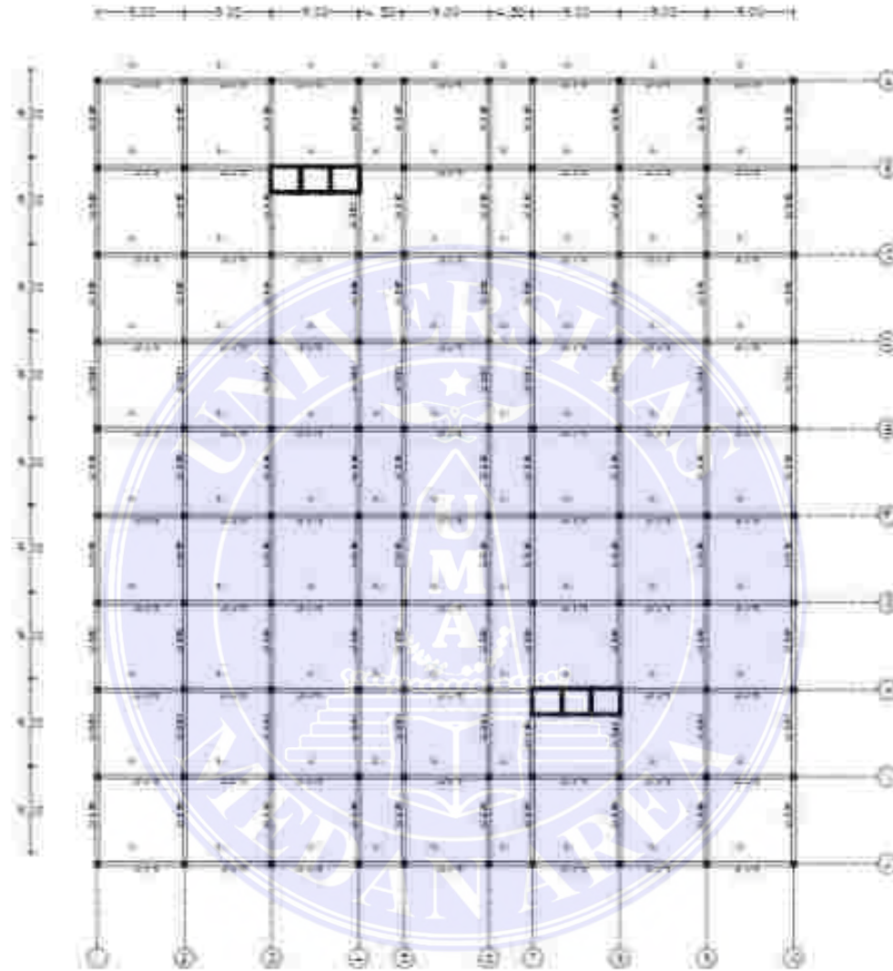
DENAH PERENCANA BLOOF SKALA 1:50
