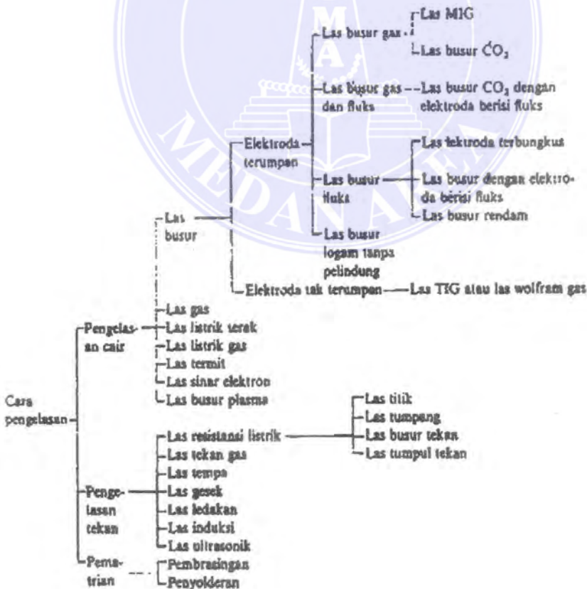
Gambar 2.1. klasifikasi pengelasan (Wirjosumarto, 2000)
