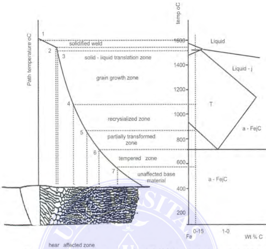
Gambar 2.11. Struktur mikro daerah HAZ pada baja karbon C \geq 0,3 \% (Easterling, 1983)
