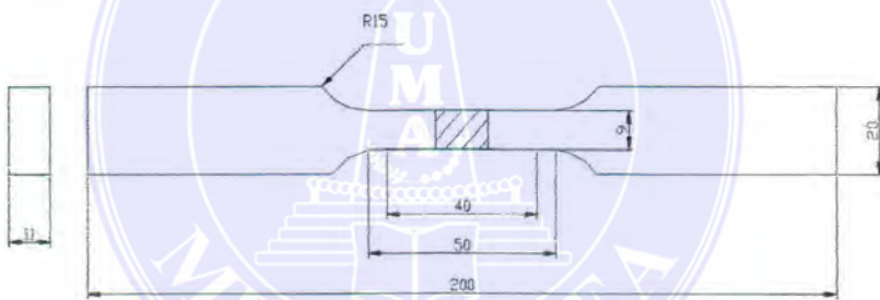
Gambar 3.8. Spesimen JIS Z 2201
