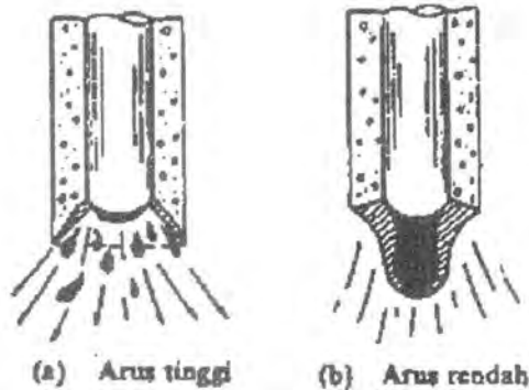
Gambar 2.3. Pemindahan logam cair
