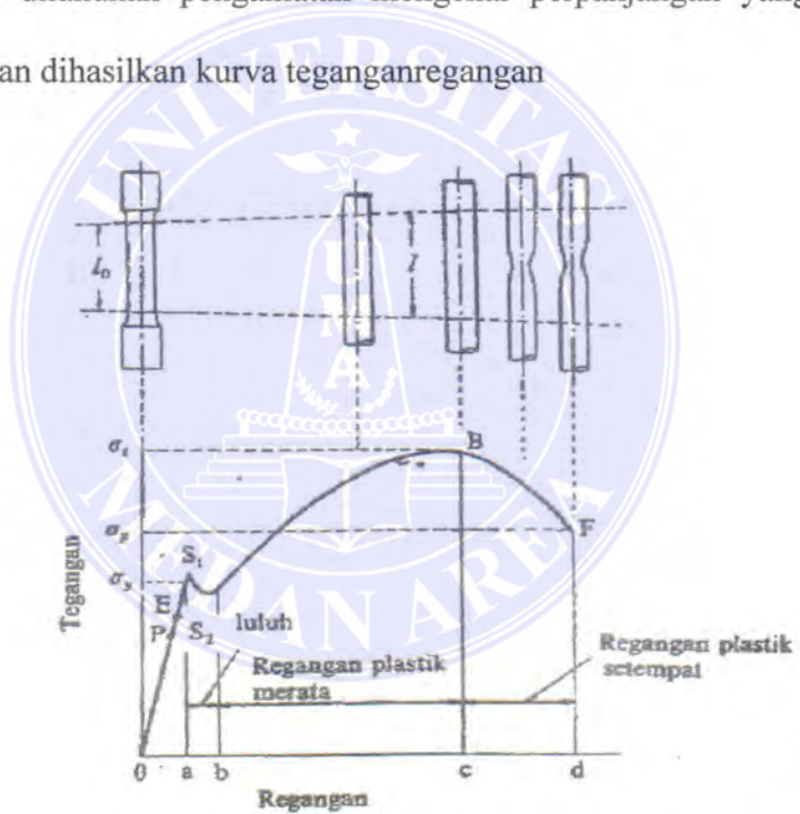
Gambar 2-21. Kurva tegangan-regangan ( Wiryosumarto, 2000)
