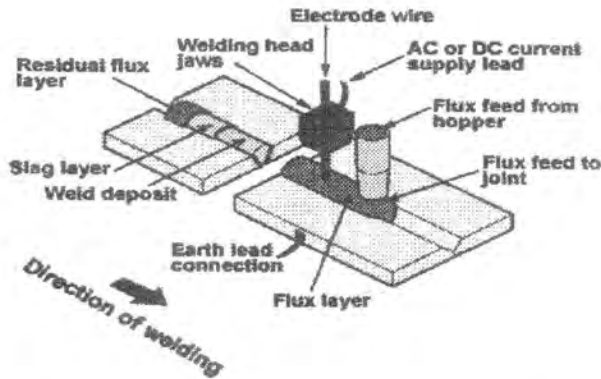
Gambar 2.9. Skema las busur logam Gas
