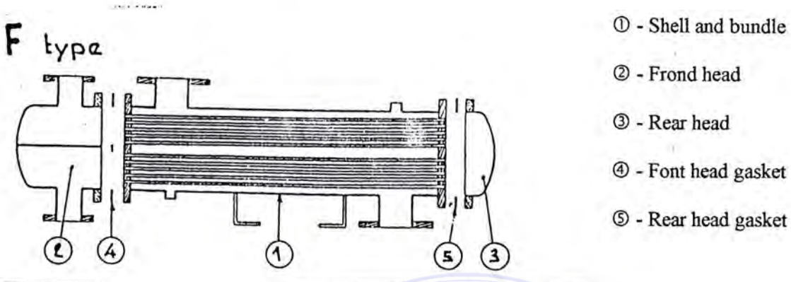
Gambar 2.10. Alat penukar kalor tipe “F”
