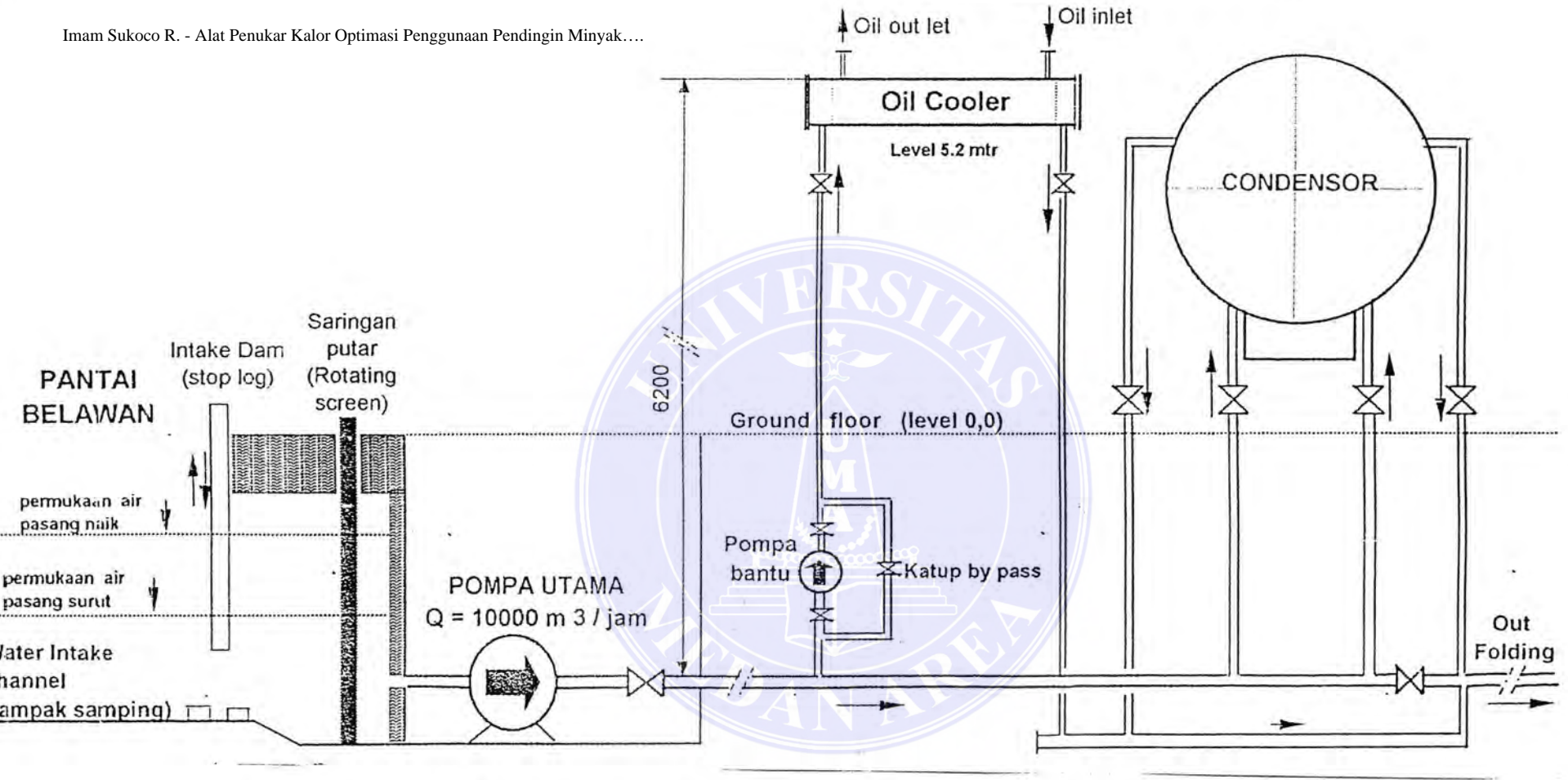
Gambar 3.1. Skets Media Pendingin dengan Pompa Bantu (Auxiliary dan Saluran By Pass) (Skets setelah modifikasi)
