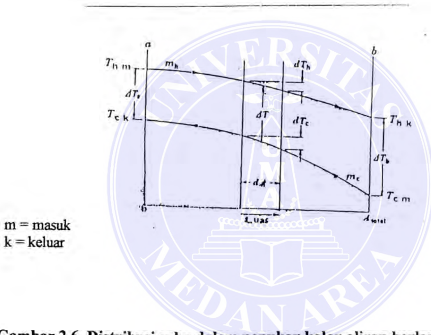
Gambar 2.6. Distribusi suhu dalam penukar kalor aliran berlawanan (Counter flow) lintas tunggal
