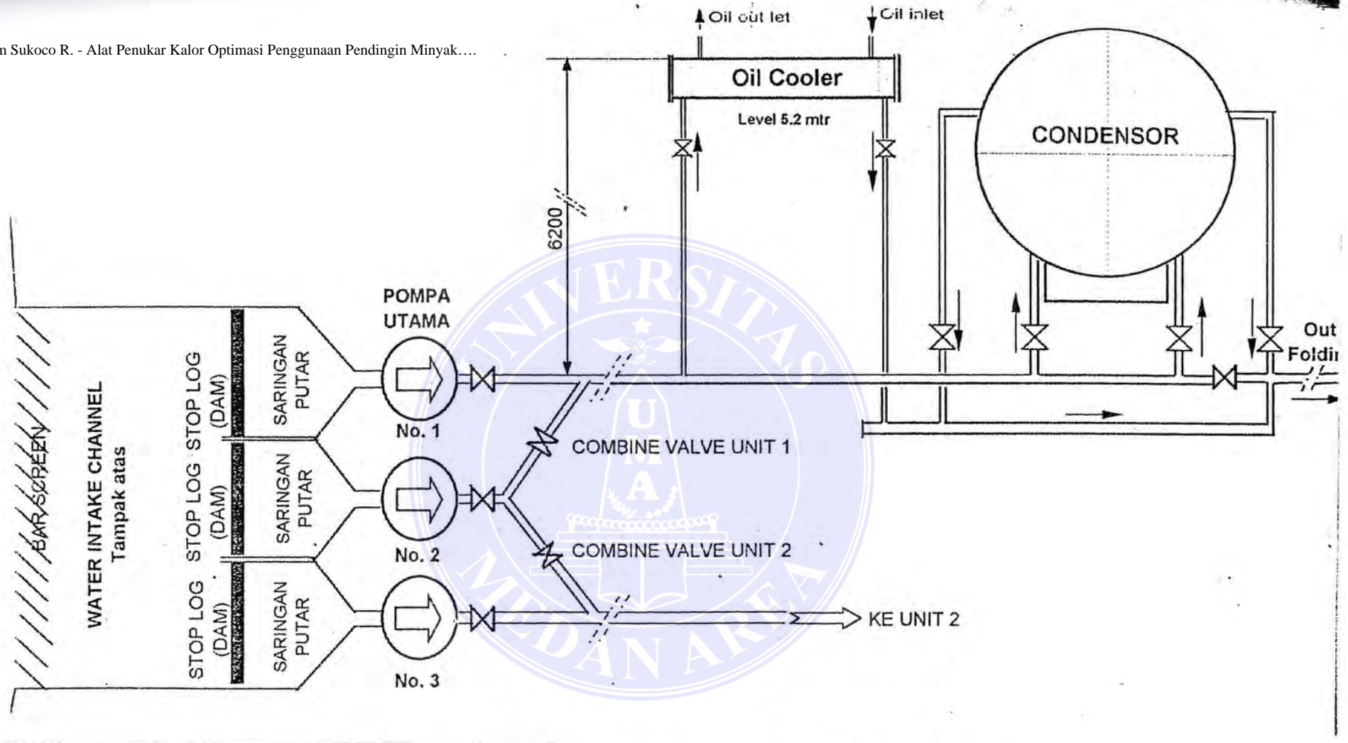
Gambar 1.1. Skets Aliran Air Pendingin ke Kondensator dan Oil Cooler (Existing)
