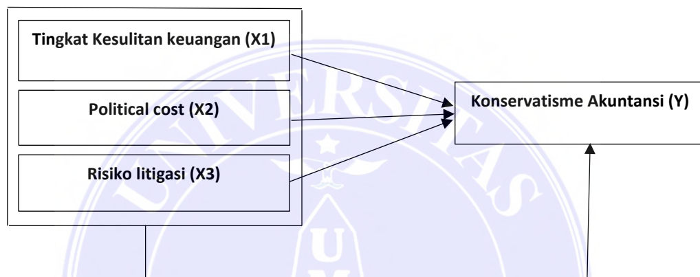
Gambar 2.1 Kerangka Pemikiran
