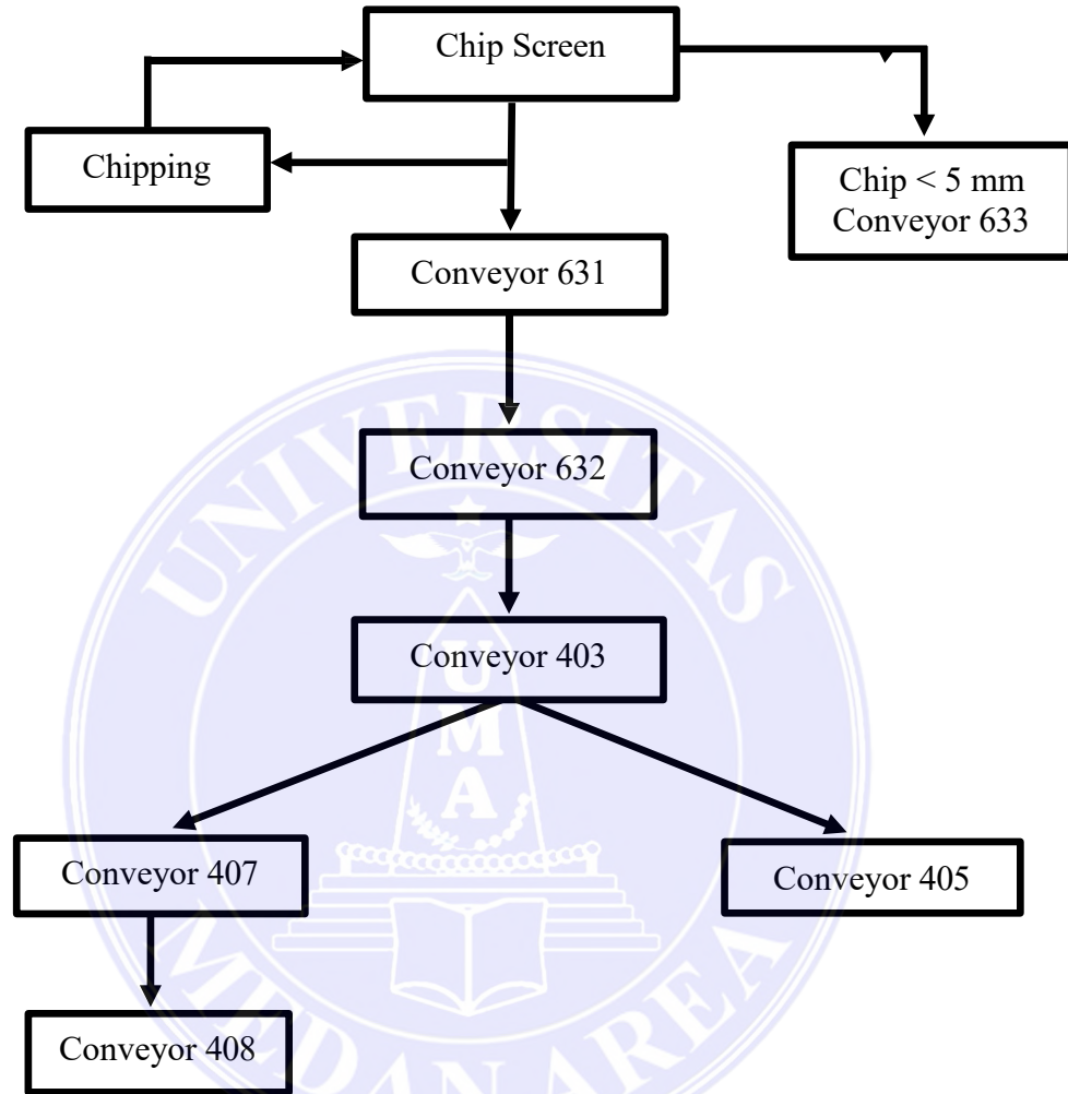
Gambar 3.23. Aliran Chip
