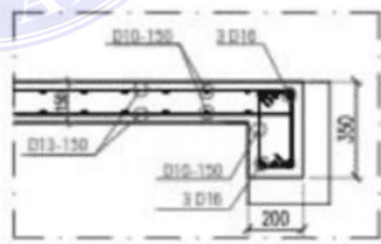
05 DETAIL 2 SKALA 1:25
