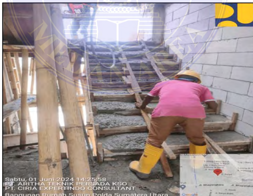
Gambar 4 Pengecoran tangga
