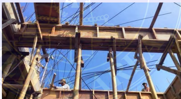
Gambar 3.1.8 Bekisting
