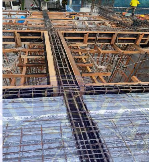
Gambar 4.4 Pemasangan Tapak Balok Sumber : Dokumentasi Proyek, 2024
