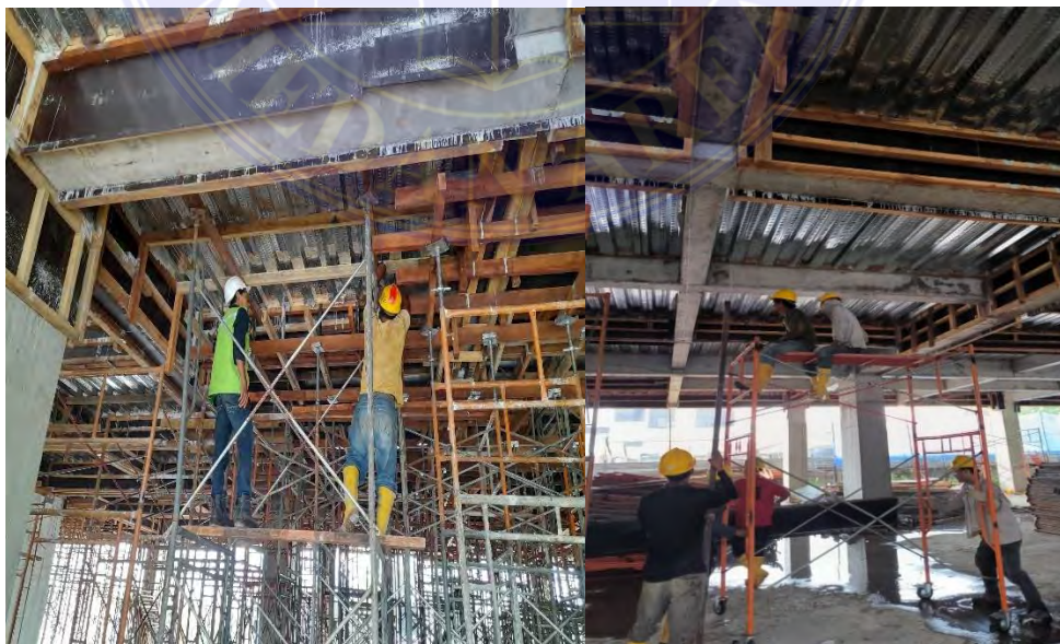
Gambar 4.11 Pelepasan Bekisting dan Perancah
