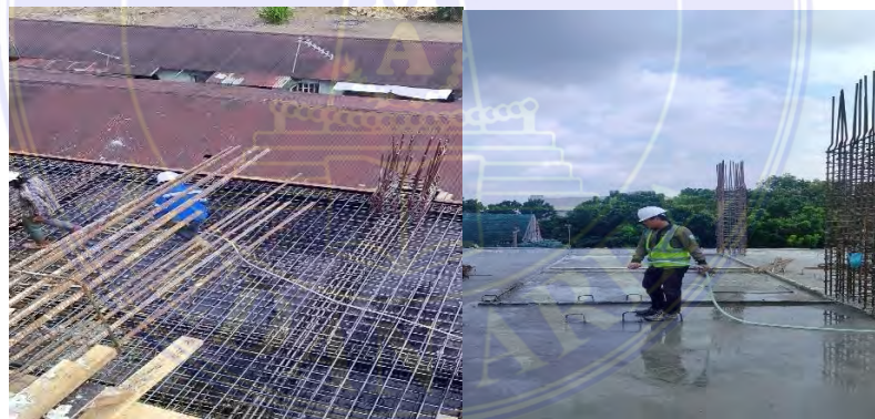
Gambar 4.7 Pembersihan Dan Perawatan Lokasi Cor Sumber : Dokumentasi Proyek, 2024
