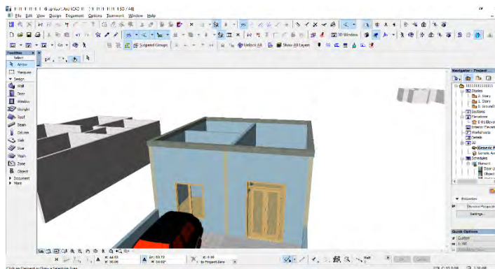
Gambar 3. 16 Pengerjaan ring balok pada archicad.
