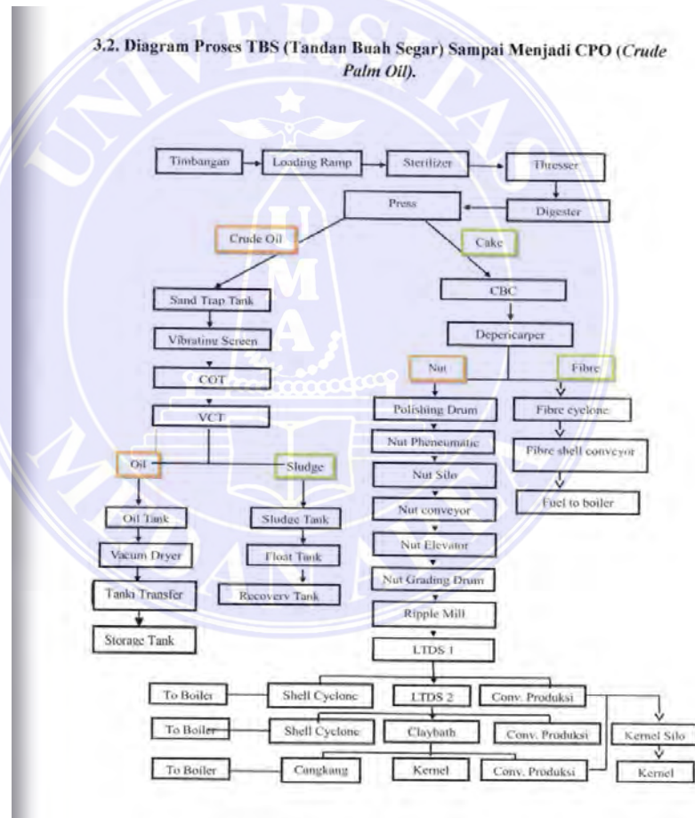
gambar 16. diagram proses TBS sampai CPO
