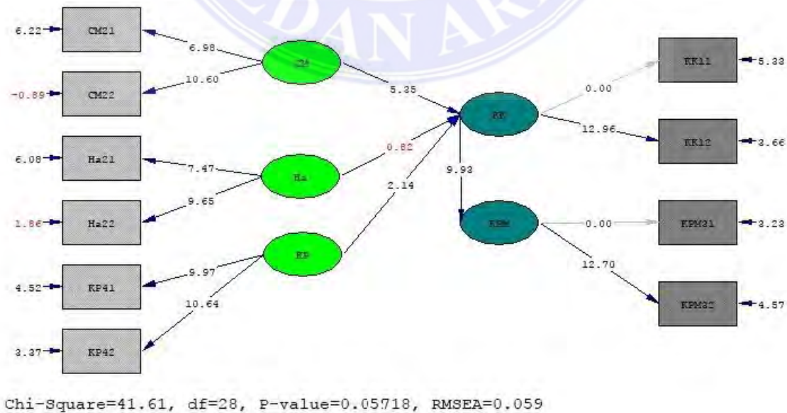
Gambar.2. Pengujian LISREL
