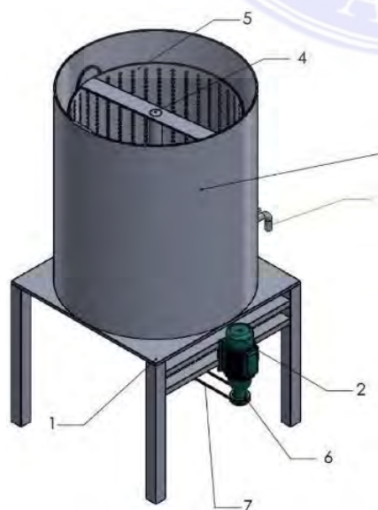
Gambar 1. Desain mesin peniris keripik pisang
