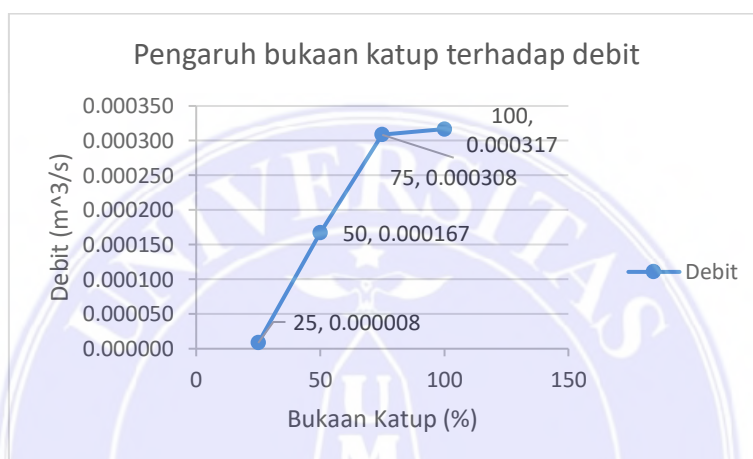
Gambar 14. Pengaruh bukaan katup terhadap debit air
