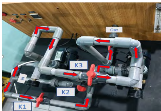
Gambar 11. Susunan instalasi pompa paralel
