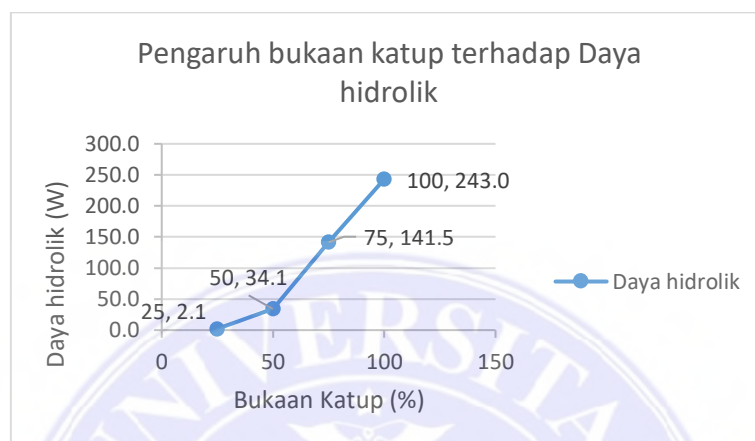
Gambar 16. Pengaruh bukaan katup terhadap daya hidrolik
