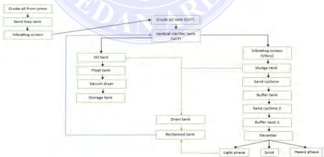
Gambar 3. 16 Alur Proses Klarifikasi
