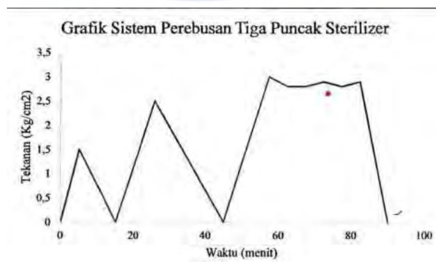
Gambar 3. 7 Grafik Perebusan
