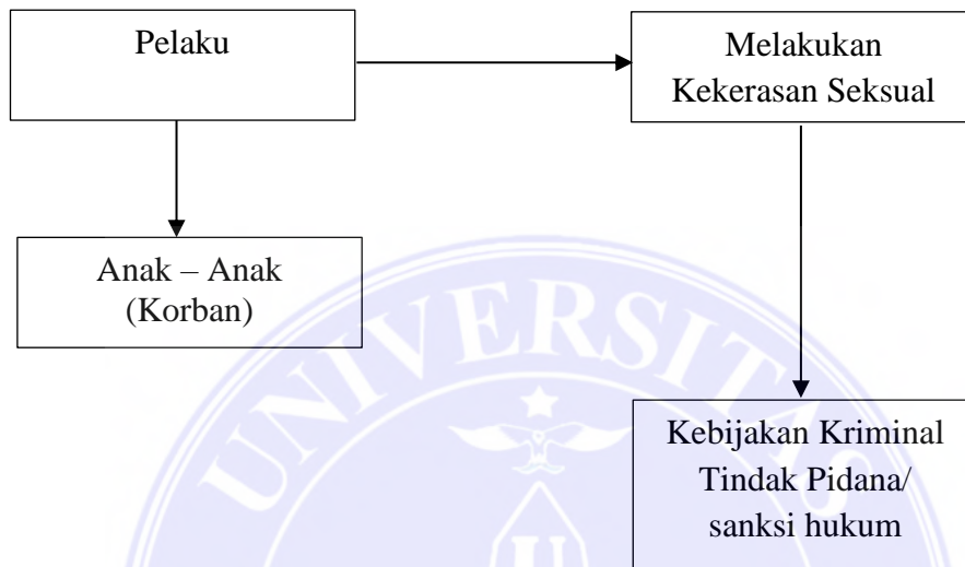
Gambar 2.1 Kerangka Berfikir
