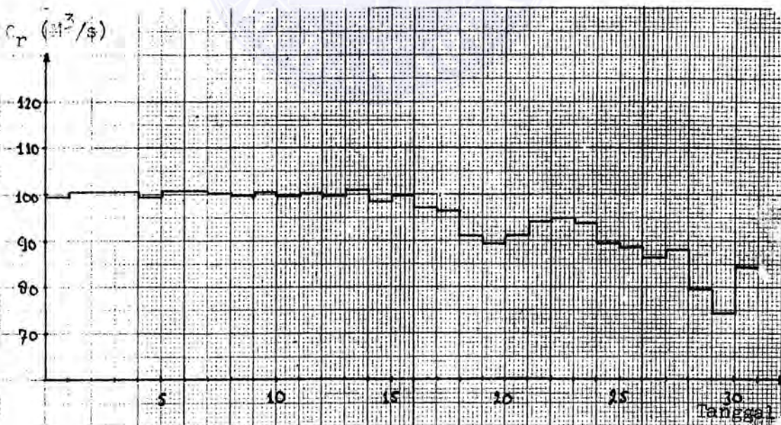
Grafik Debit Air Yang Diberikan ( Q_r )
