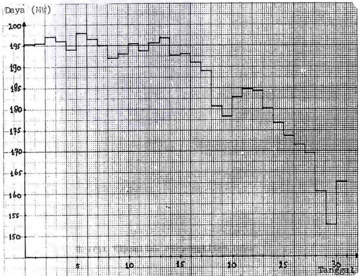
Grafik Kapasitas Pembangkitan Daya
