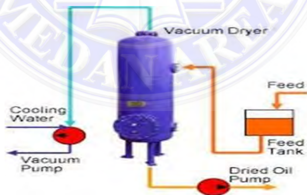
Gambar 3. 28. Bagian Bagian Vacuum Dryer
