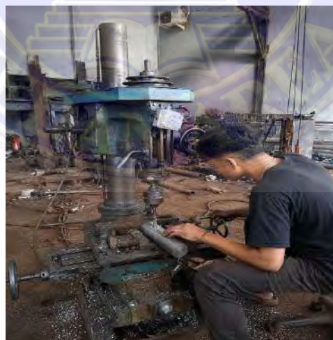
Gambar 3.30 Melakukan pengeboran
