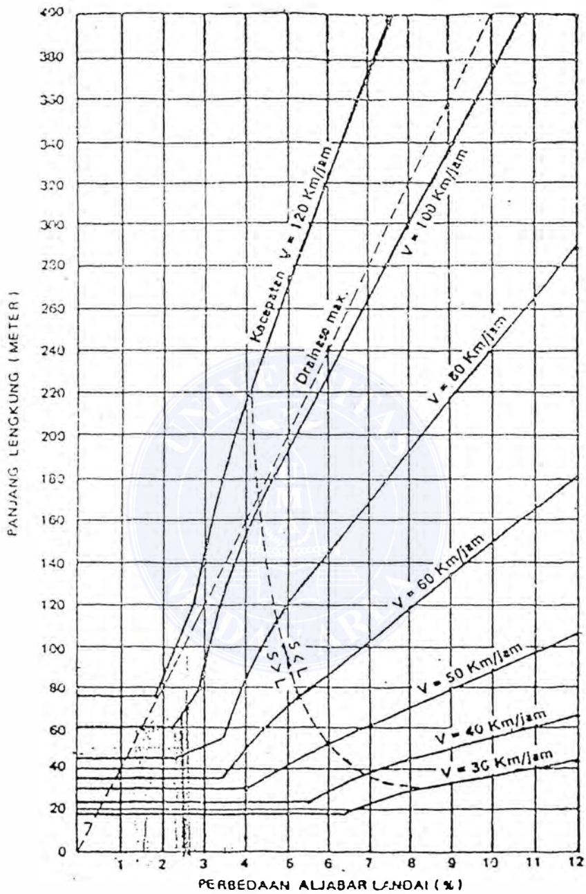
2.2 GRAFIK V. PANJANG LINGKUNG VERTIKAL CEKUNG
