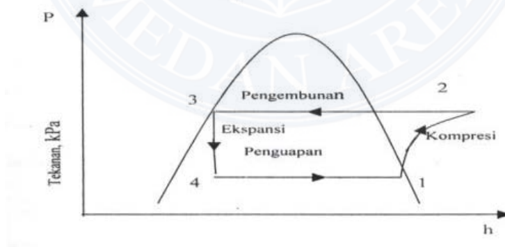
Gambar 2.8 Diagram tekanan entalpi siklus kompresi uap standar.
