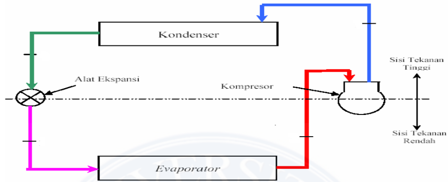
Gambar 2.10 Sistem refrigerasi kompresi uap
