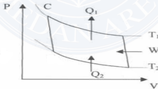
Gambar 2.7 siklus refrigerasi carnot
