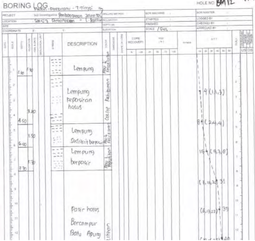
Gambar: Bore Hole Typical Tanah di BM-12 Sta. 42+ 950
