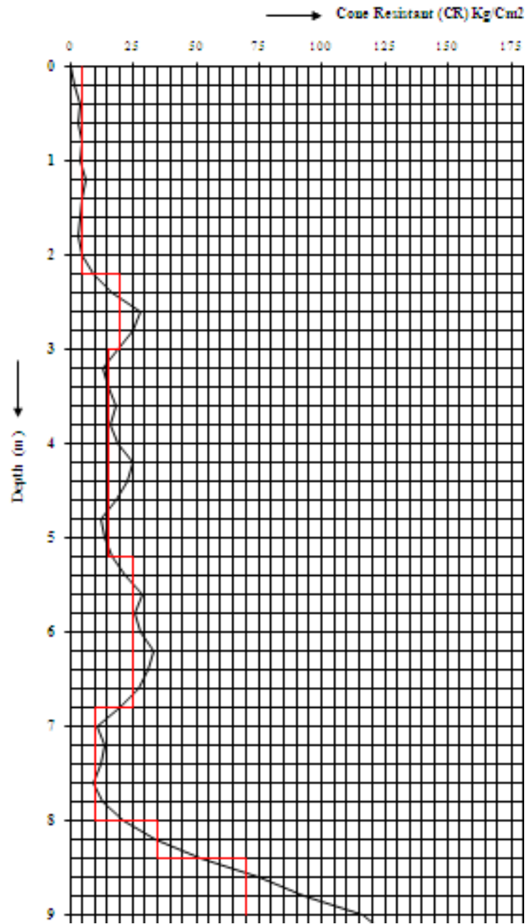
Gambar: Kondisi lapisan tanah pada titik sondir 9, Sta 2+000
