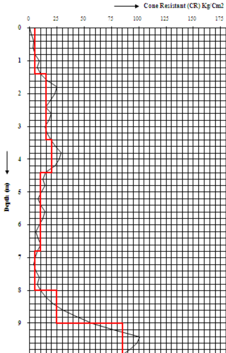
Gambar: Kondisi lapisan tanah pada titik sondir 8, Sta 1+900
