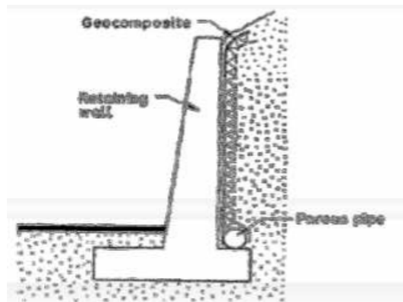
Gambar 2.10 Drainase Sumber: Departemen P.U., 2009
