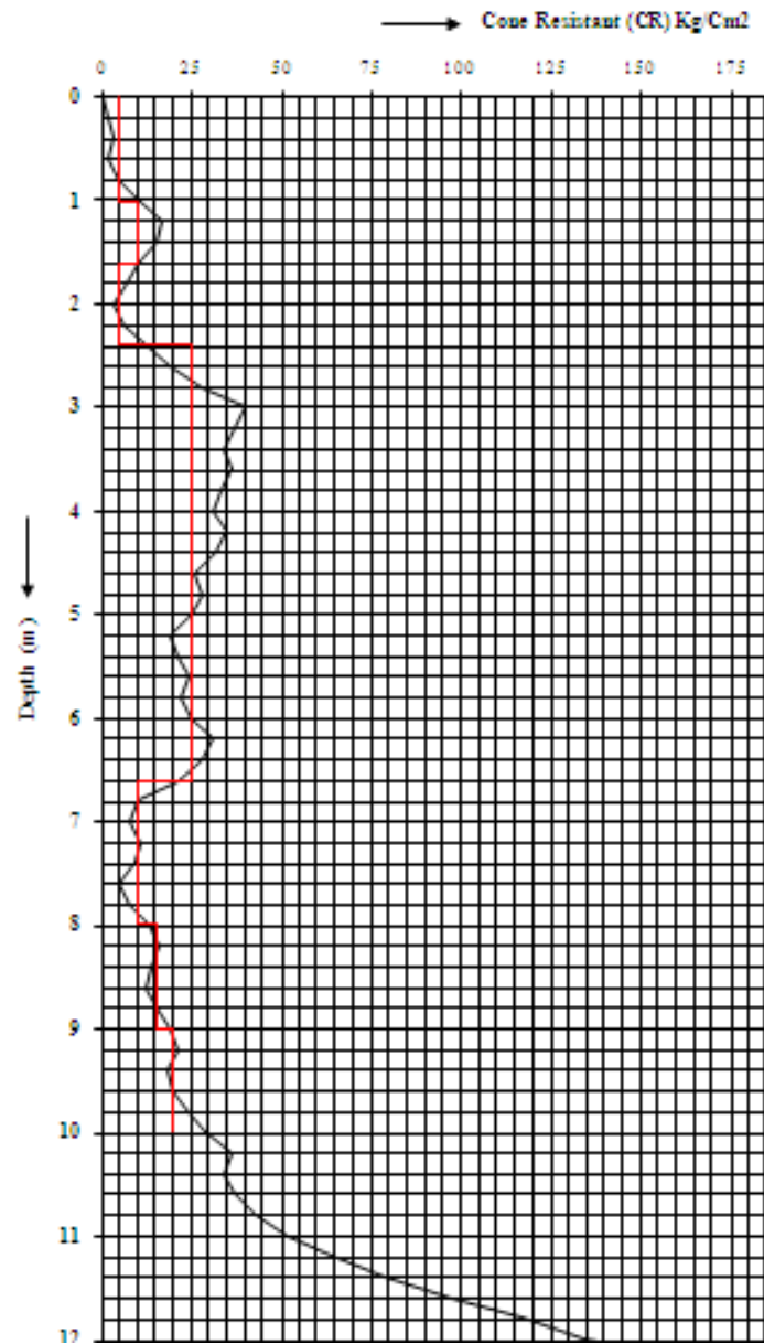
Gambar: Kondisi lapisan tanah pada titik sondir 2, Sta 0+650
