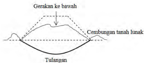
c. Keruntuhan menyeluruh tanah pondasi
