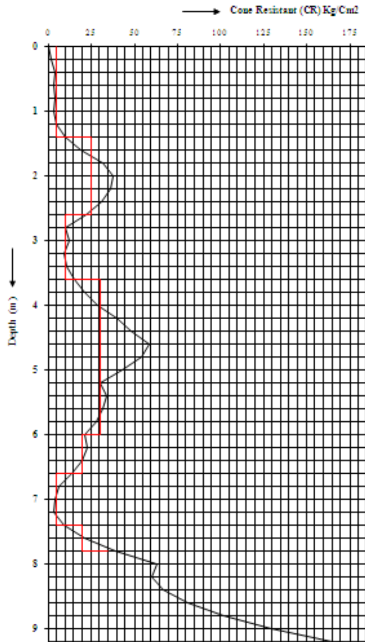
Gambar: Kondisi lapisan tanah pada titik sondir 10,Sta 2+100
