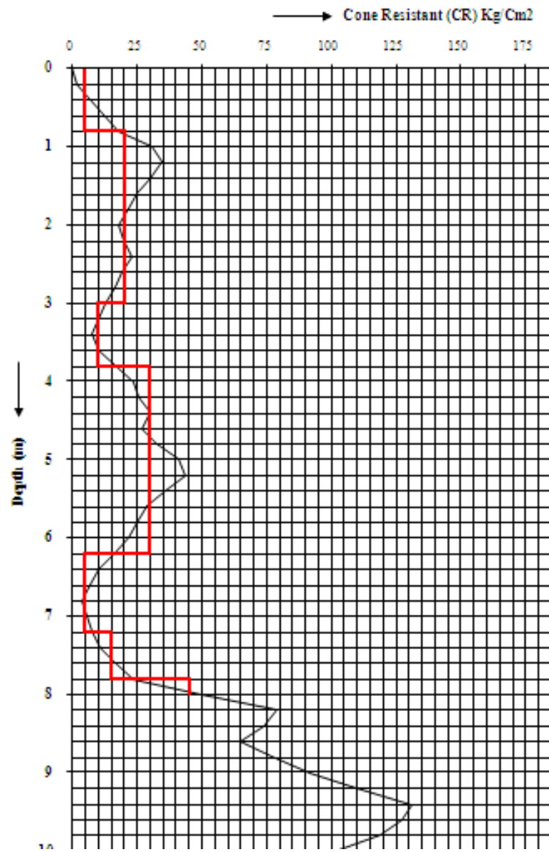
Gambar: Kondisi lapisan tanah pada titik sondir 6,Sta 1+650
